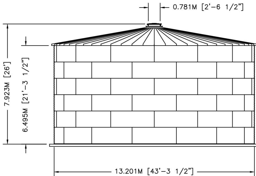
ELEVATION
